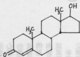
圖一：睪丸酮
